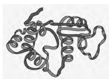
opgevouwen eiwitmolecuul
