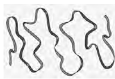
uitgevouwen eiwitmolecuul
